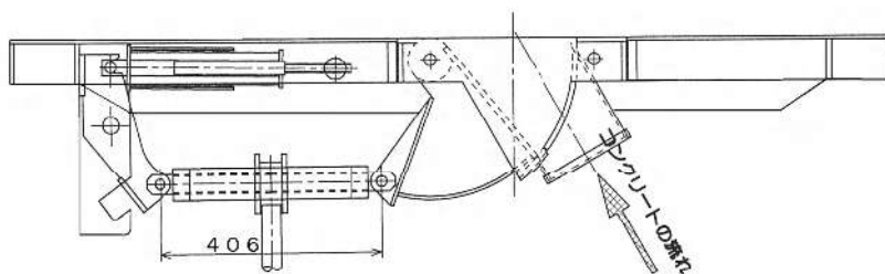
図-2 ゲート<開>の状態
